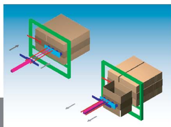
APERTURA DEI CARTONI
